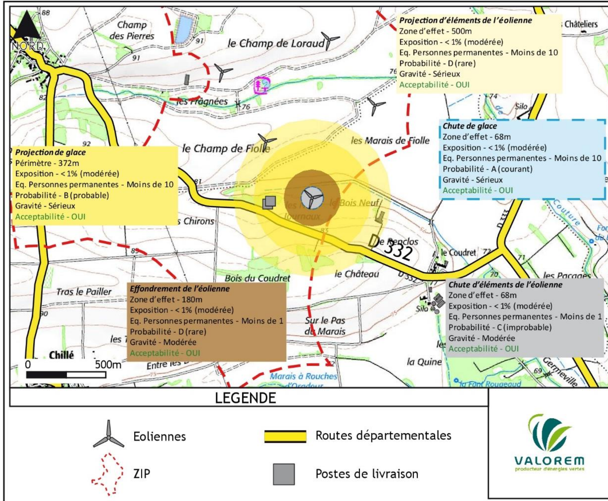
Cartographie de synthèse des risques pour l'éolienne n° 4
