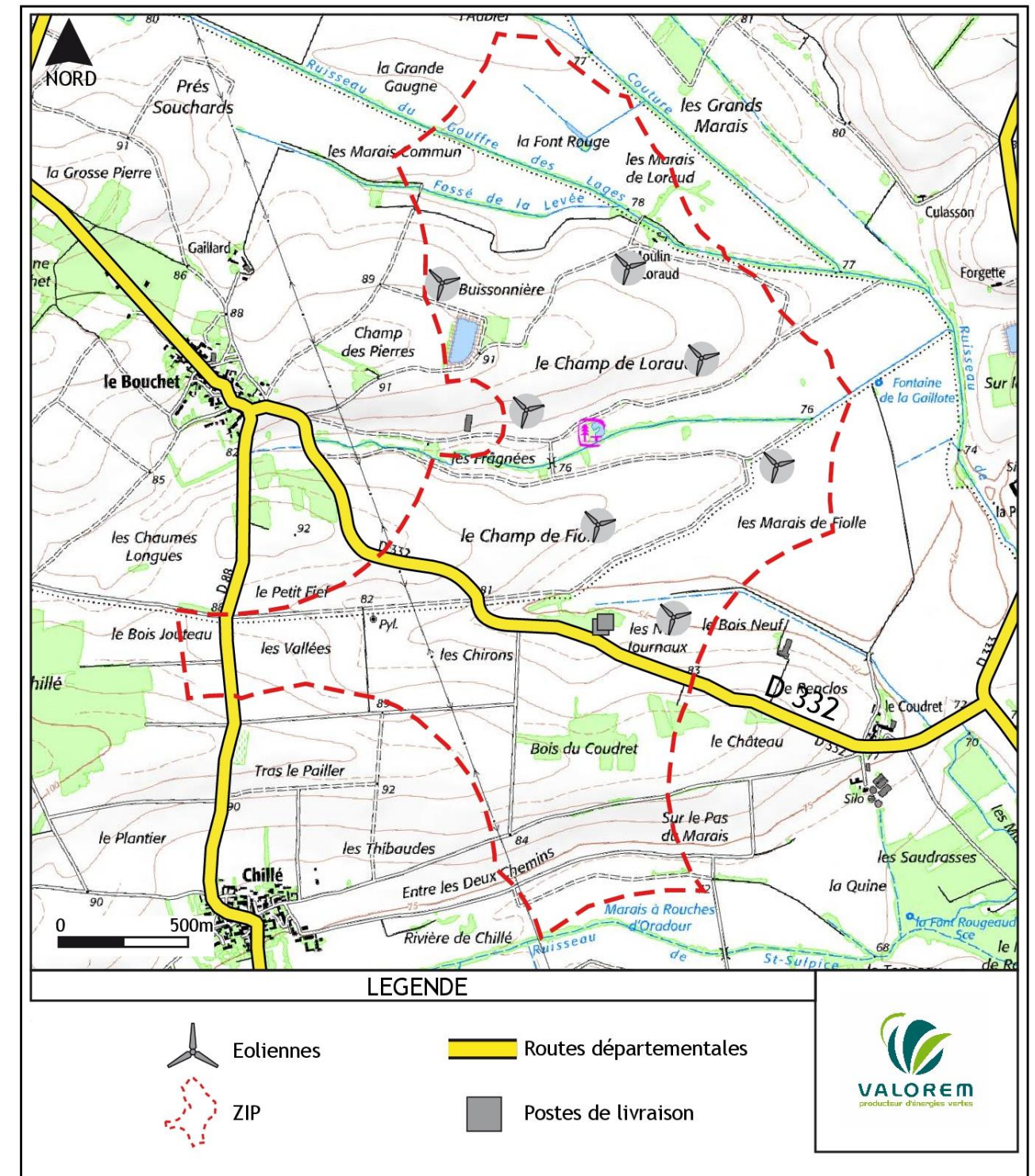
Zone d'effet du phénomène « Chute de glace »
