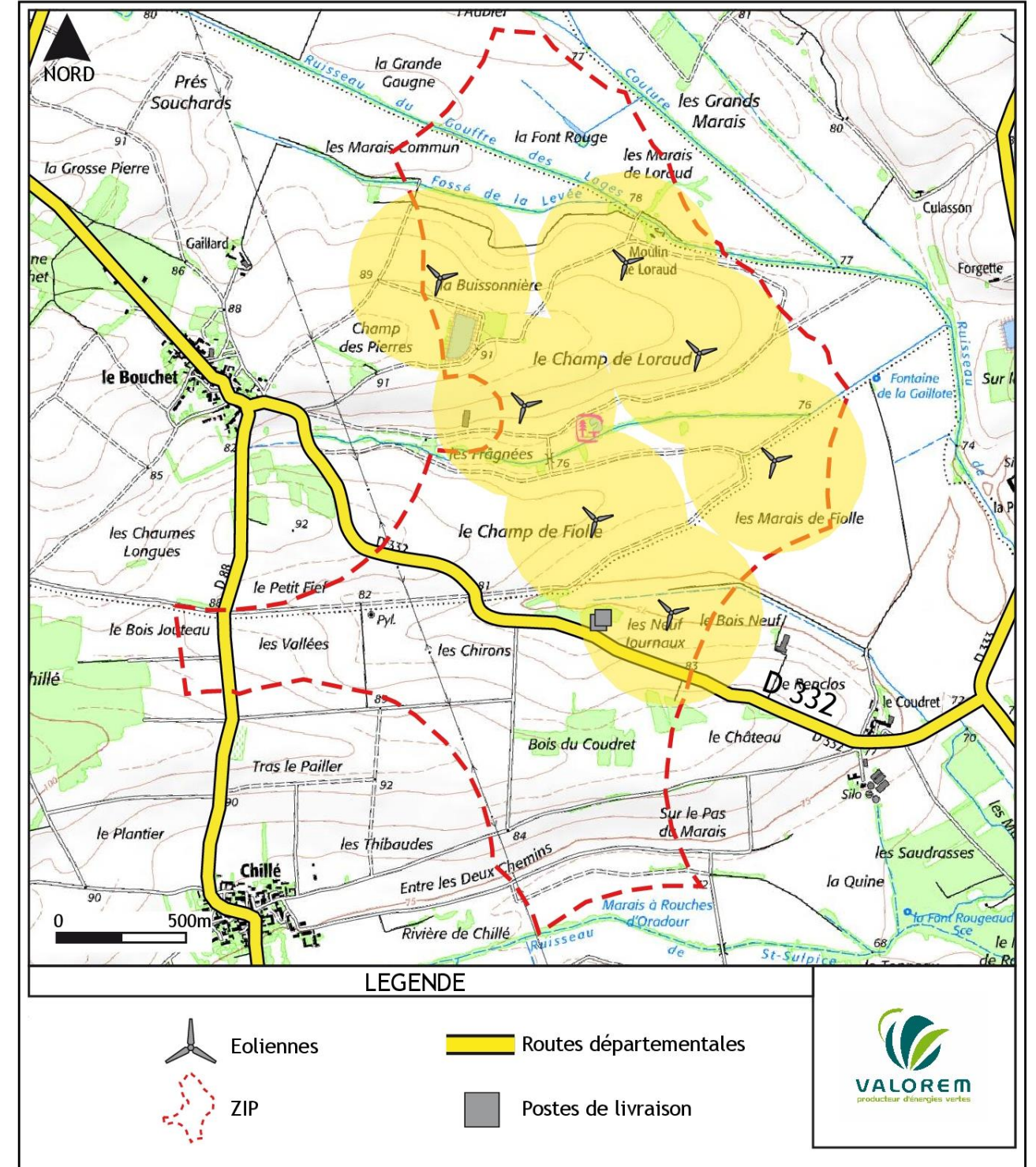
Zone d'effet du phénomène « Projection de glace » (372 m)
