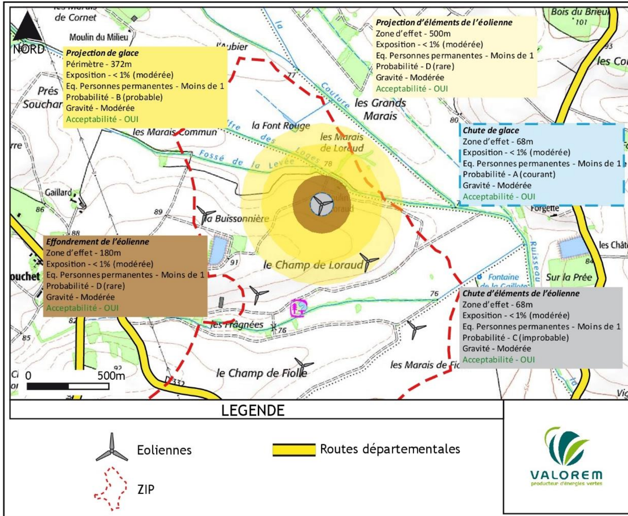
Cartographie de synthèse des risques pour l'éolienne n° 5
