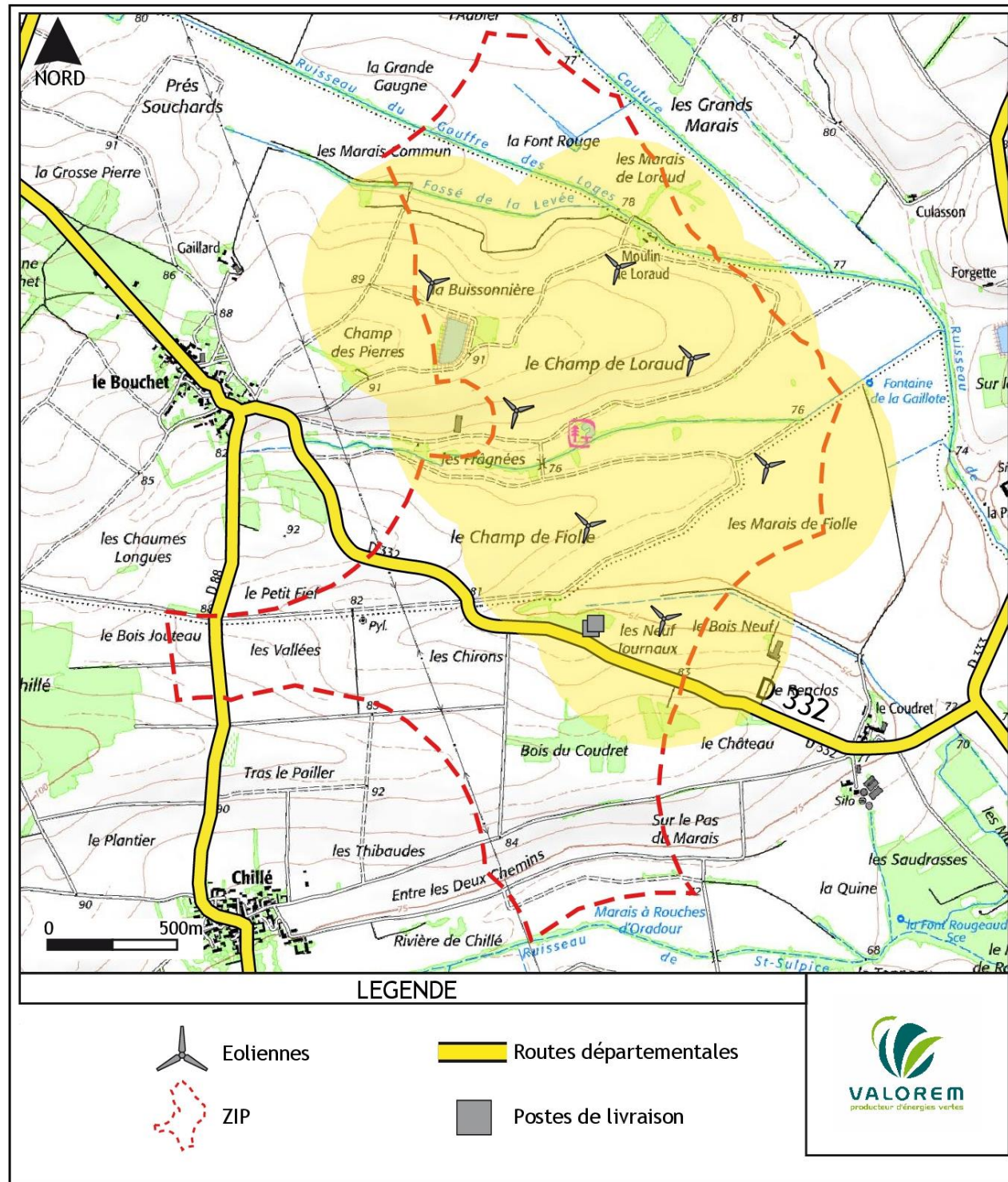
Zone d'effet du phénomène « Projection de pales ou de fragments de pales » (500 m)
