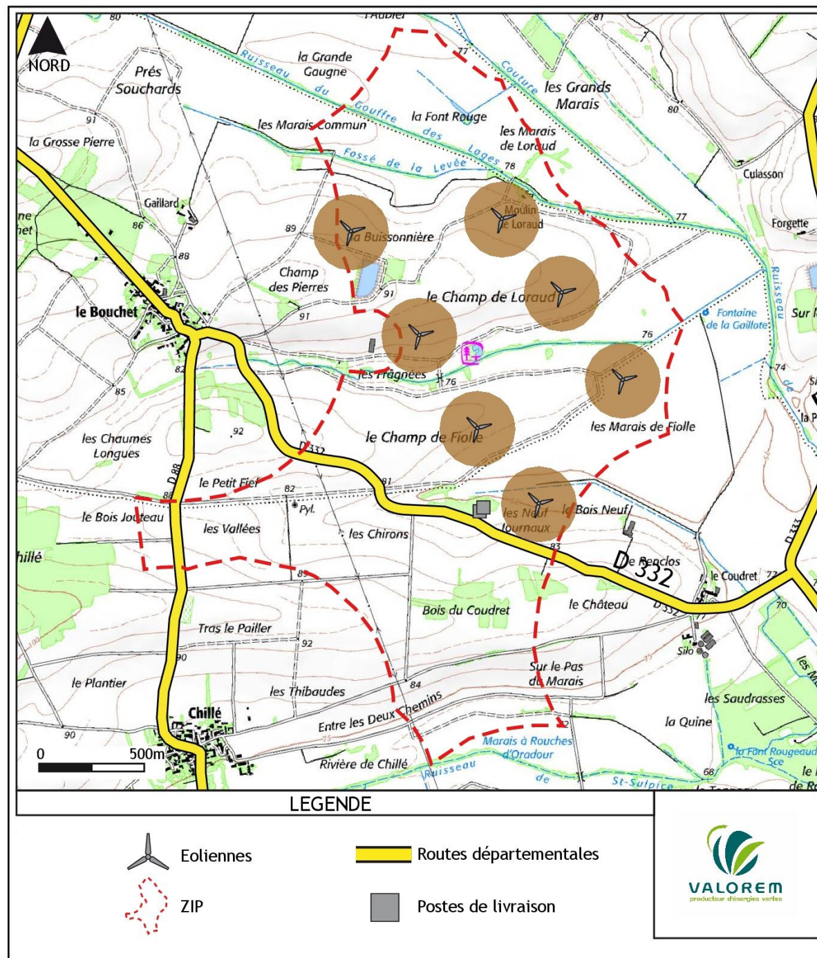
Zone d'effet du phénomène « Effondrement de l'éolienne » (180 m)
