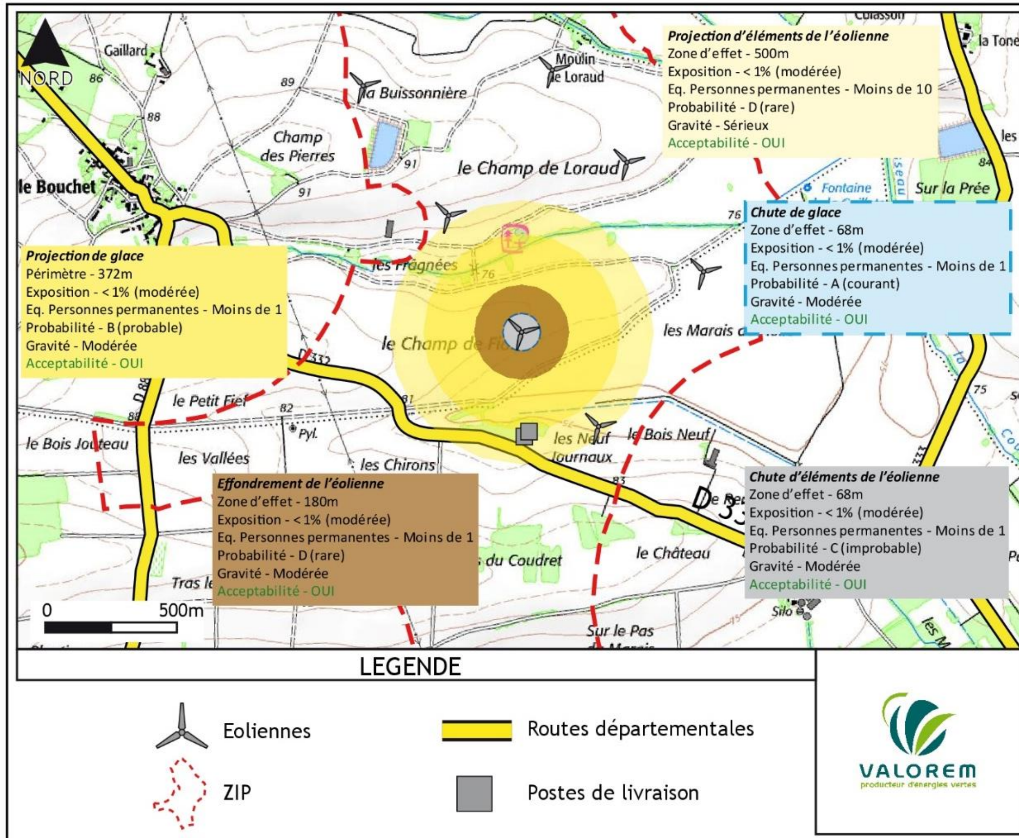
Cartographie de synthèse des risques pour l'éolienne n° 3
