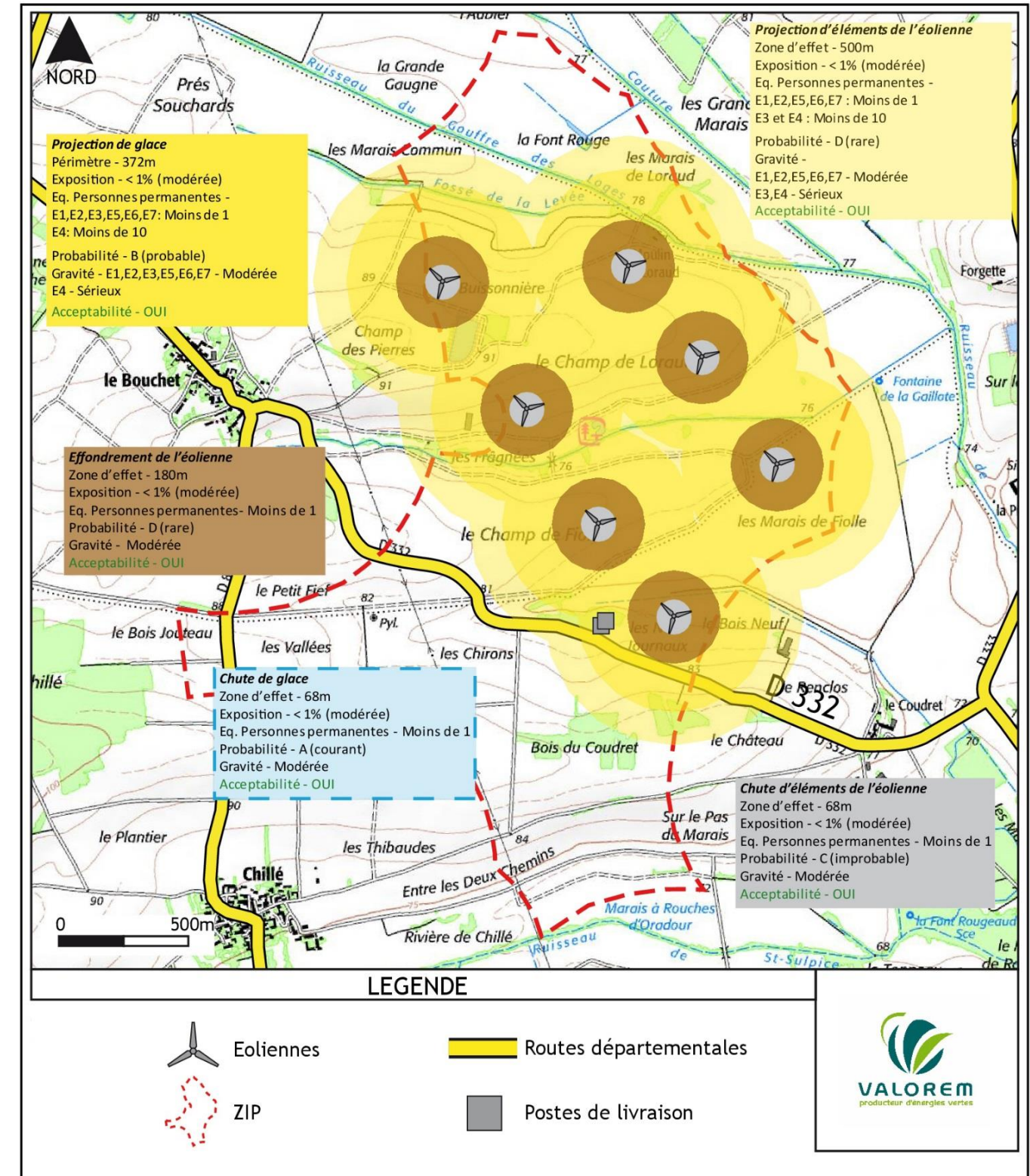
Cartographie de synthèse des risques pour le projet éolien de la Couture
