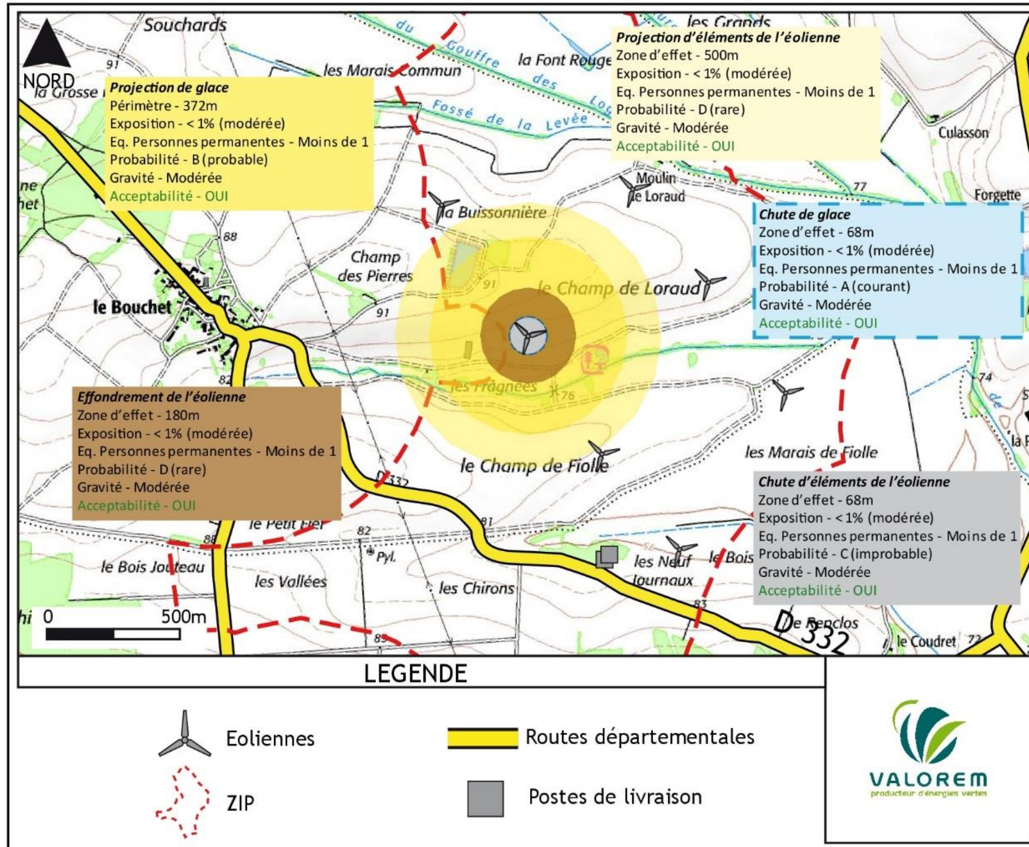
Cartographie de synthèse des risques pour l'éolienne n° 2
