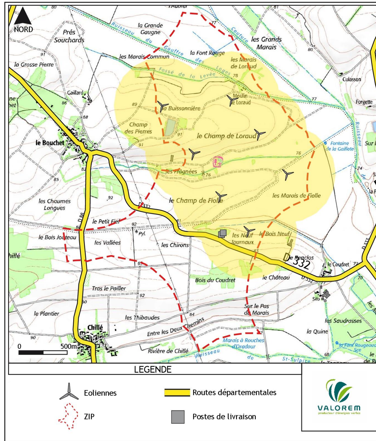
Zone d'effet du phénomène « Projection de pales ou de fragments de pales »
