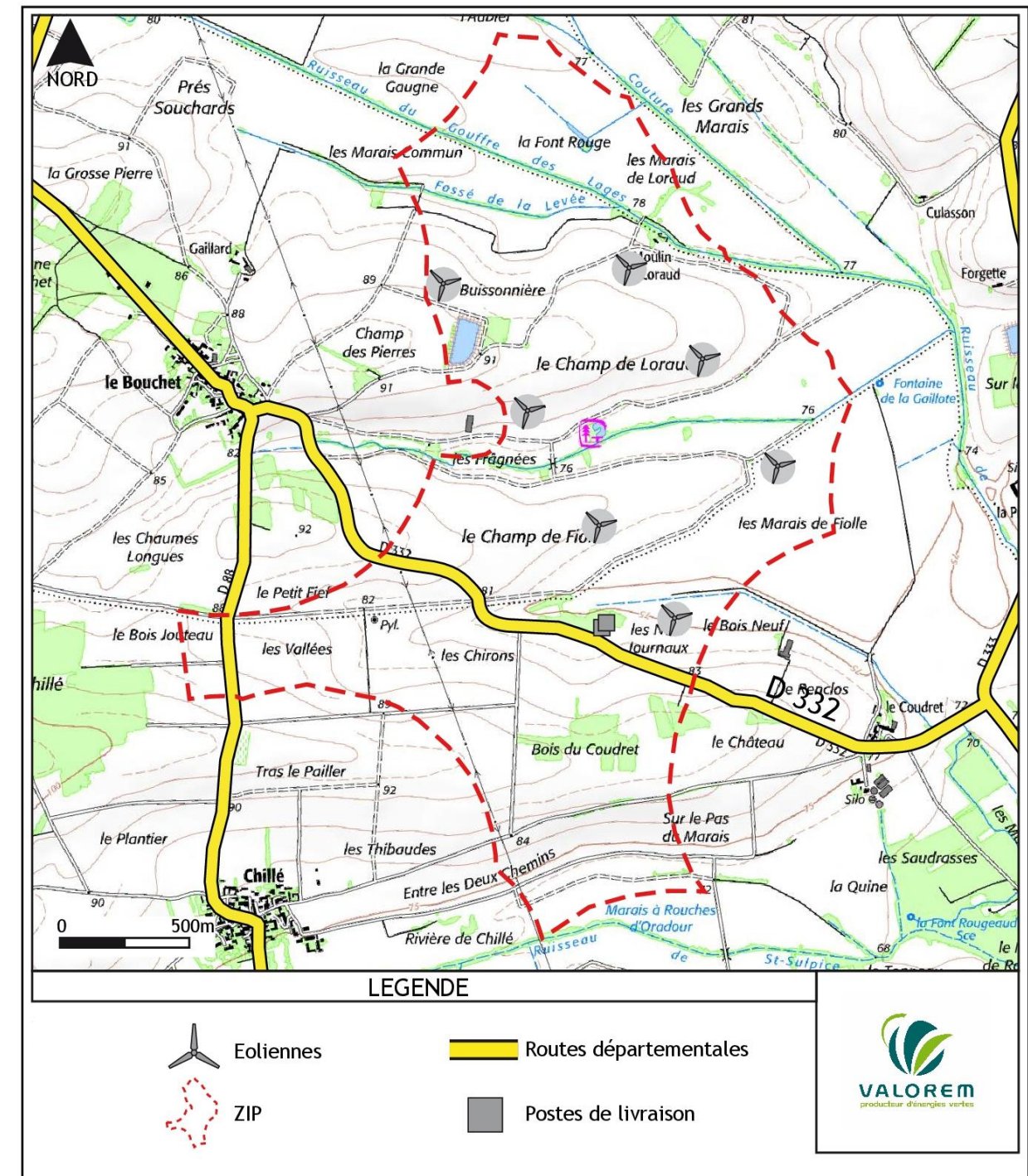
Zones d'effet des phénomènes « Chute de glace » et « Chute d'éléments de l'éolienne » (68 m)
