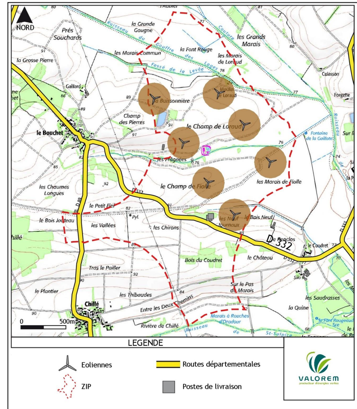
Zone d'effet du phénomène « Effondrement de l'éolienne »
