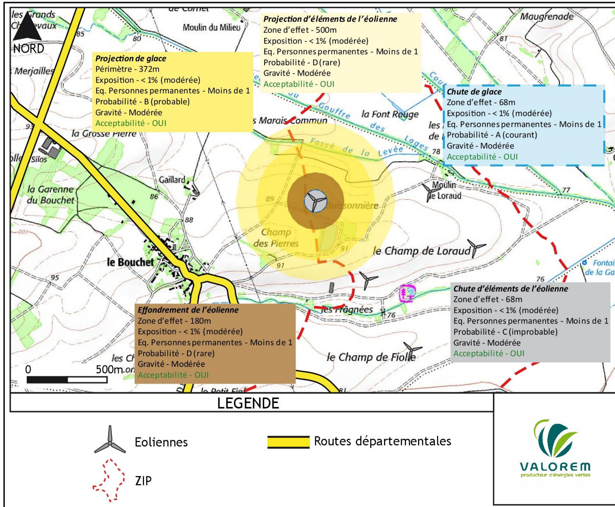
Cartographie de synthèse des risques pour l'éolienne n° 1
