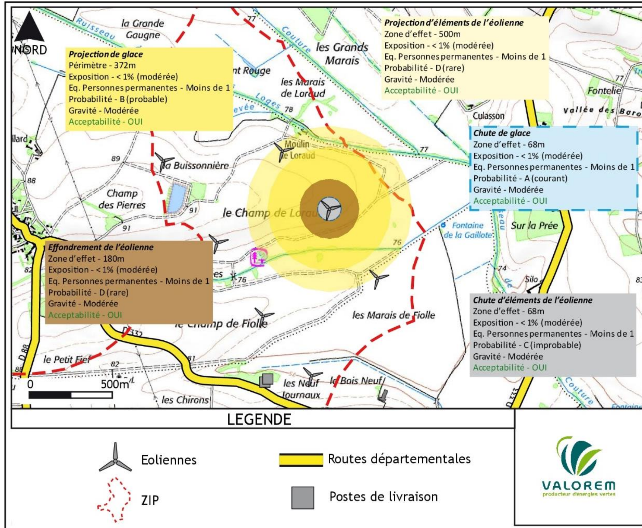
Cartographie de synthèse des risques pour l'éolienne n° 6
