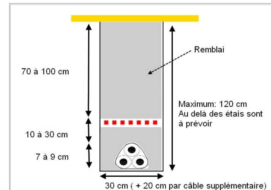
Coupe de tranchée pour enfouissement de ligne
