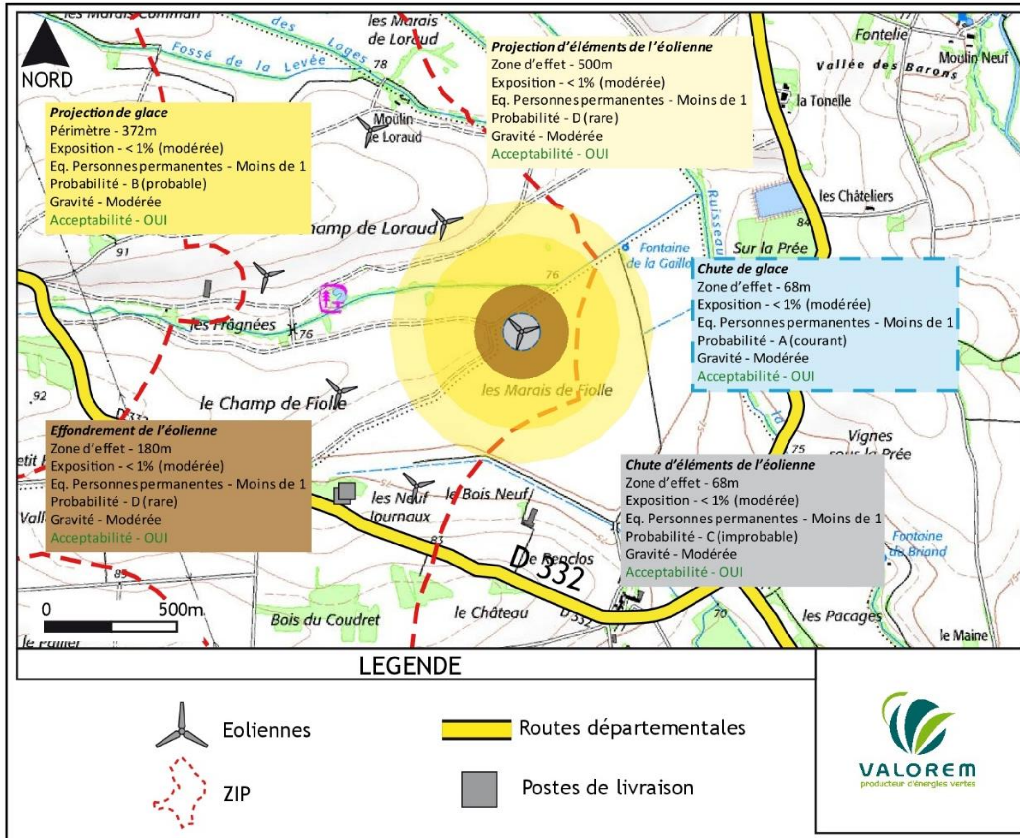
Cartographie de synthèse des risques pour l'éolienne n°7
